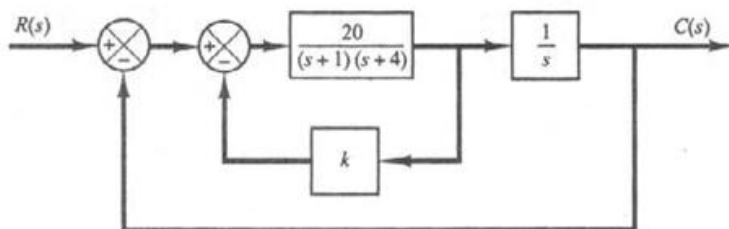
شکل ۶-۶ سیستم کنترل.
