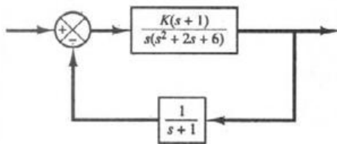
شکل ۶-۱۰۱ سیستم کنترل.
