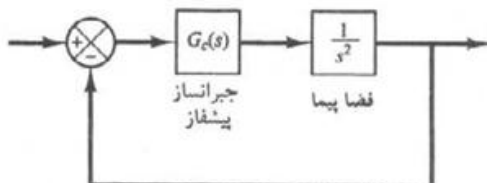
شکل ۱۰۸-۶ سیستم کنترل.
