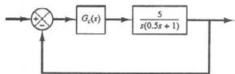
شکل ۱۰۷-۶ سیستم کنترل.
