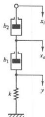
شکل ۷۴-۶ سیستم مکانیکی.
