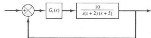
شکل ۱۱۱-۶ سیستم کنترل.
