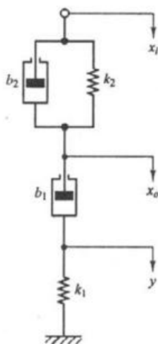
شکل ۷۵-۶ سیستم مکانیکی.
