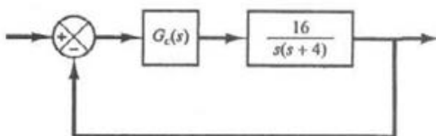
شکل ۱۰۹-۶ سیستم کنترل.
