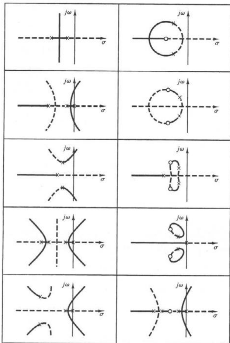
جدول ۲-۶ مکان هندسی ریشه‌ها برای سیستمهای دارای فیدبک منفی و فیدبک مثبت.
