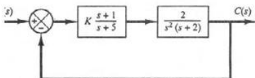
شکل ۶-۱۰۰ سیستم کنترل.
