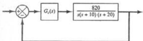
شکل ۱۱۰-۶ سیستم کنترل.
