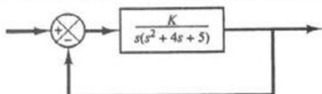
شکل ۶-۱۰۴ سیستم کنترل.
