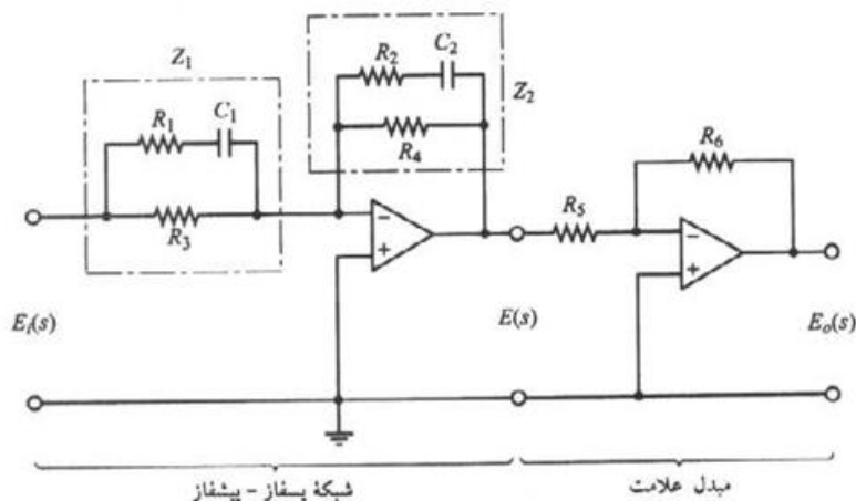
شکل ۶-۵۳ جبران‌ساز پسفاز - پیشفاز.
