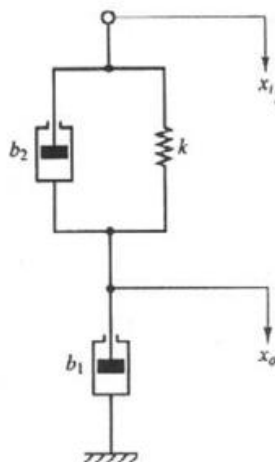
شکل ۶-۱۰۳ سیستم مکانیکی.
