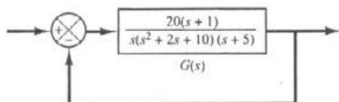
شکل ۷-۱۶۲ سیستم کنترل.
