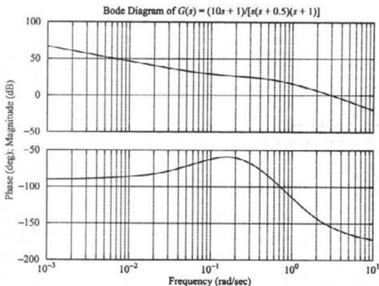
شکل ۷-۱۳۹ نمودار بوده G(s) = (10s + 1)/[s(s + 0.5)(s + 1)] .
