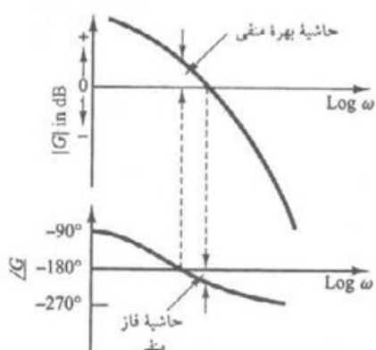
سیستم ناپایدار
