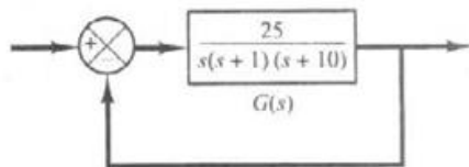
شکل ۷-۱۶۱ سیستم کنترل.
