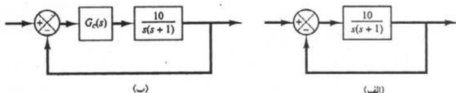
شکل ۷-۱۴۴ (الف) سیستم کنترل؛ (ب) سیستم جبران شده.
