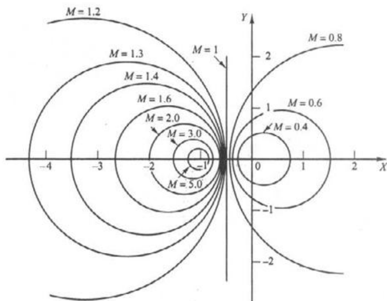
شکل ۸۱-۷ دست‌ای از دایره‌های M ثابت.
