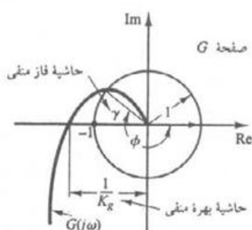
سیستم ناپایدار
