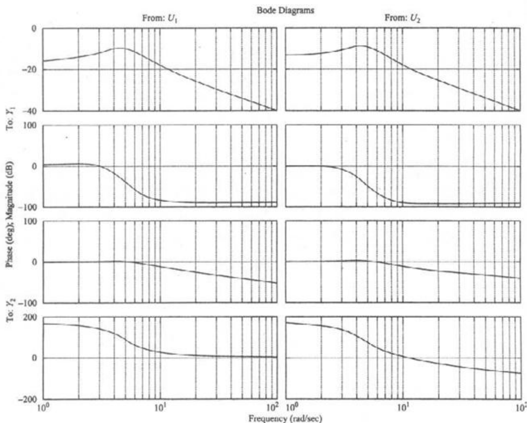
شکل ۱۱۹-۷ نمودارهای بوده .
