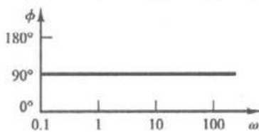
نمودار بودی G(j\omega) = j\omega
