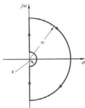
شکل ۷-۱۵۶ مسیر نایکویست
