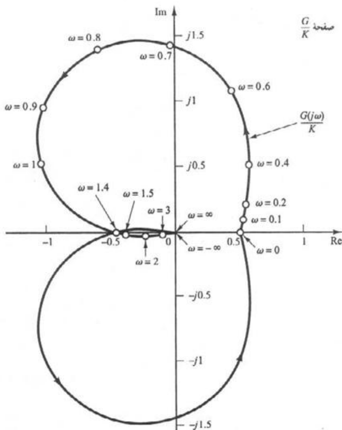
شکل ۶۱-۷ نمودار قطبی G(j\omega)/K .
