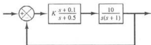
شکل ۷-۱۶۳ سیستم کنترل.
