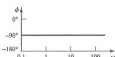
نمودار بودی G(j\omega) = 1/j\omega
