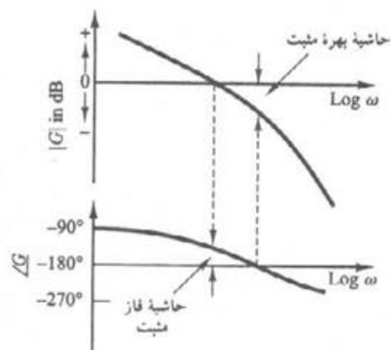
سیستم پایدار
