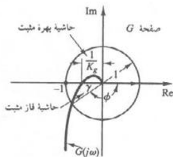
سیستم پایدار
