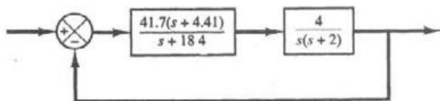
شکل ۷-۹۷ سیستم جبران شده.
