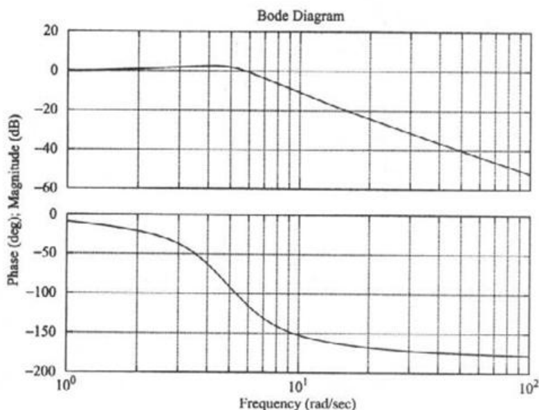
شکل ۲۴-۷ نمودار بوده سیستم مثال ۷-۷.
