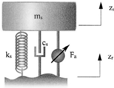
Figure 10-6. Sprung mass mode
