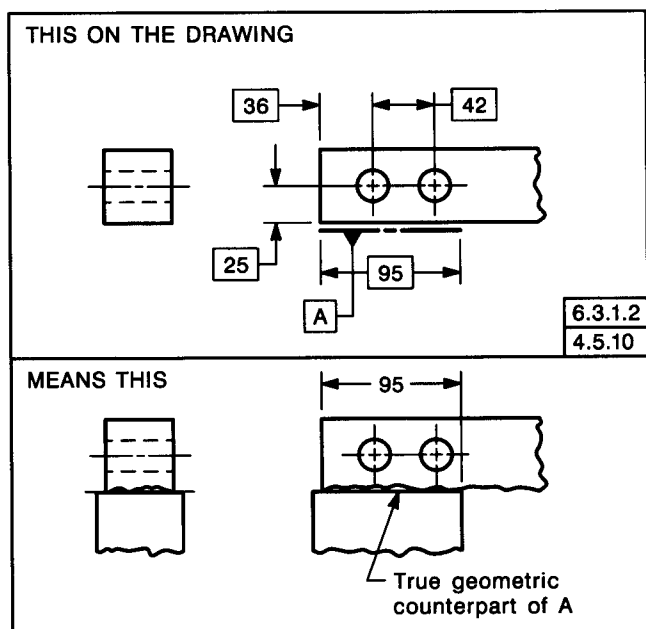
FIG. 4-23 PARTIAL DATUM
