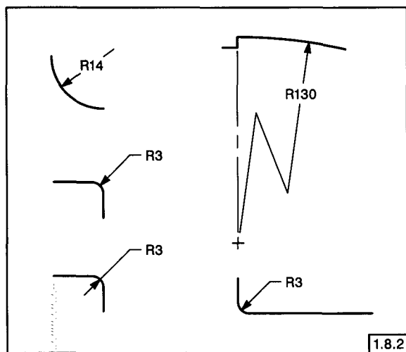
FIG. 1-20 RADII
