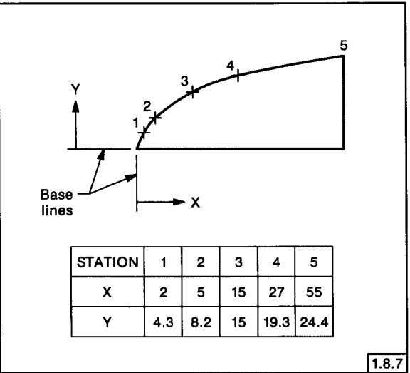
FIG. 1-32 TABULATED OUTLINE
