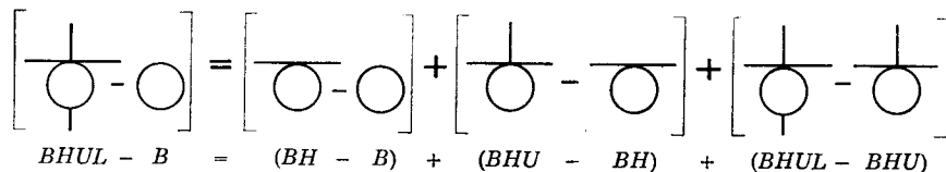
FIG. 10-23. Decomposition of empennage.
