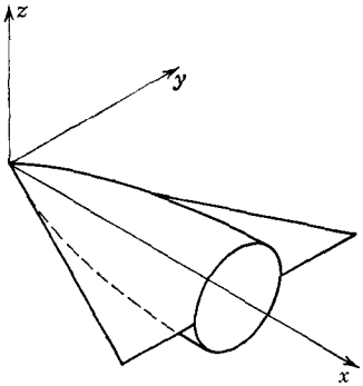
FIG. 1-1. Body axes.
