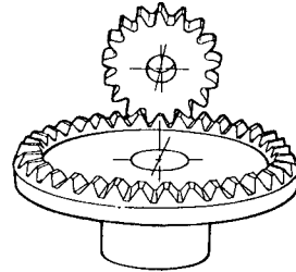
Fig. 2-19 Face Gear
