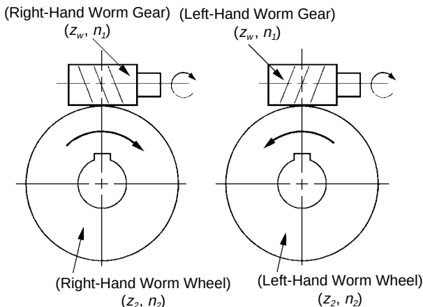
(d) Worm Mesh
