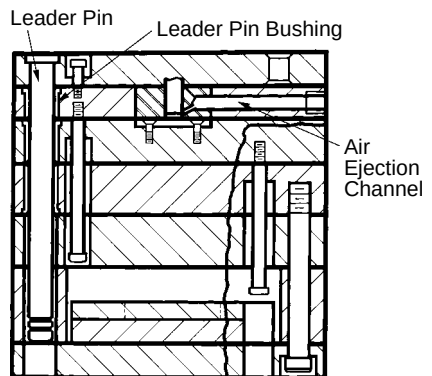
Fig. 18-10 Mold Nomenclature
