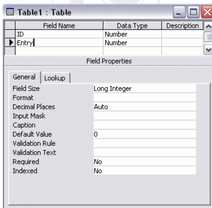
شکل ۹ - طراحی جدول جدید در اکسس.
