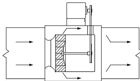
Fig. 9 Tubular Centrifugal (Inline) Fan
