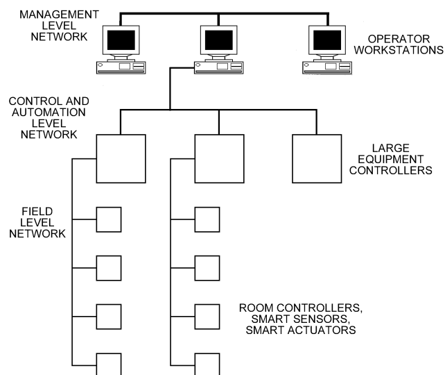
Fig. 24 Hierarchical Network
