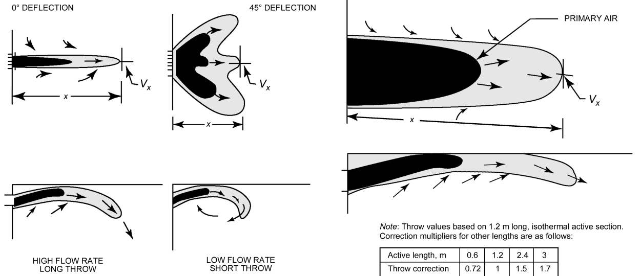
A. HIGH SIDEWALL GRILLES
