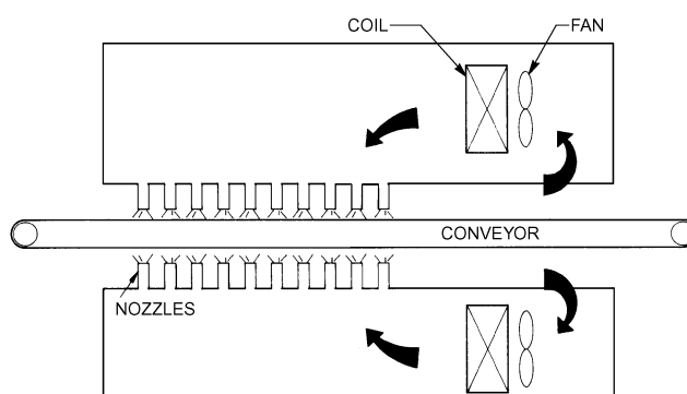
Fig. 10 Impingement Freezer
