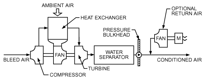
SIMPLE/BOOTSTRAP CYCLE
