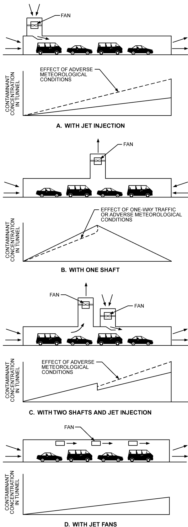
Fig. 3 Longitudinal Ventilation
