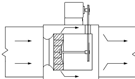
Fig. 33 Tubular Centrifugal (Inline) Fan
