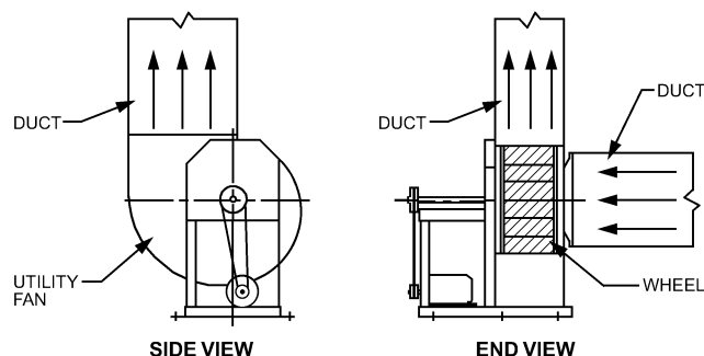
Fig. 32 Centrifugal Fan (Utility Set)
