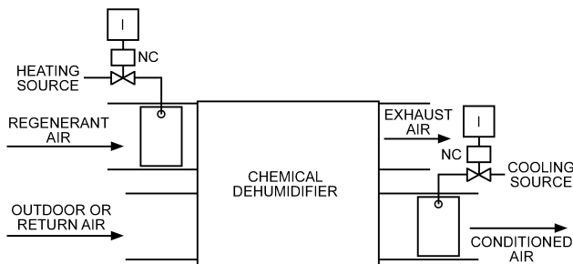
Fig. 35 Desiccant Dehumidifier
