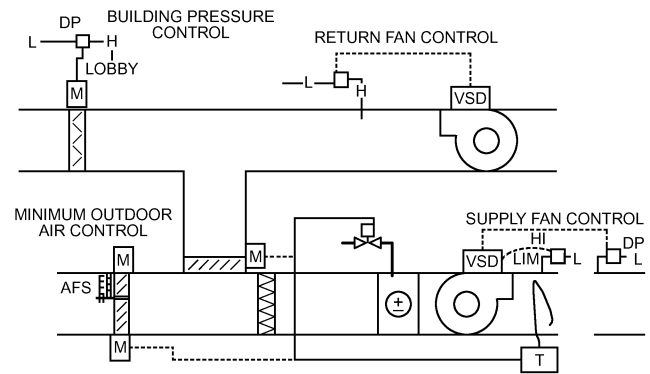
Fig. 16 Supply/Return Fan Control
