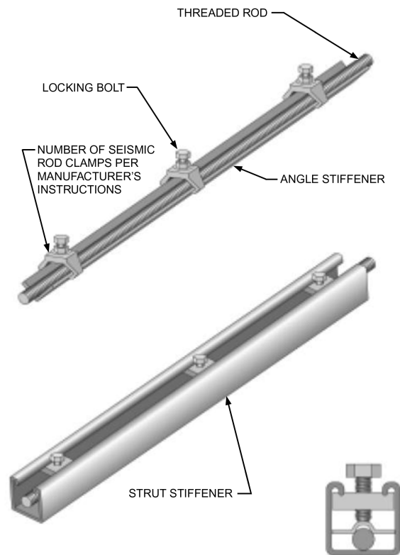
Fig. 4 Rod Stiffener
