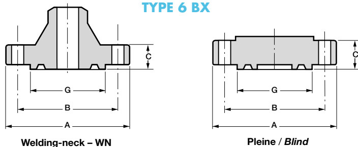
Welding-neck – WN Dia. alésage à préciser par l'acheteur / Dia. of counterbore to be specified by purchaser.
