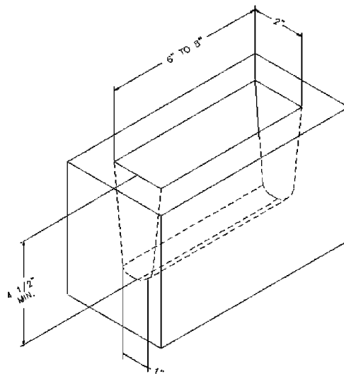
FIG. 5 b Open Keel Block Test Bar
