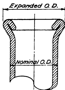
FIG. 1 Double Flare
