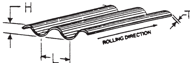
FIG. 4 Longitudinal Corrugation
