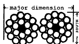
FIG. 1 Dimensions
