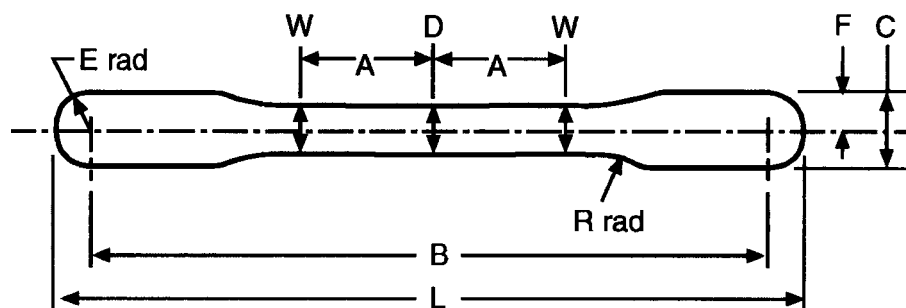
Die Dimensions
