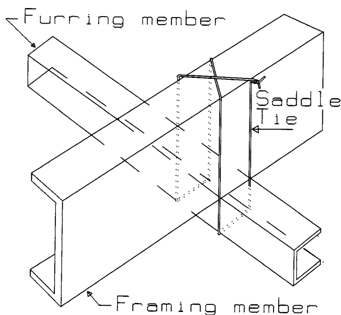
FIG. 2 Saddle-Tie
