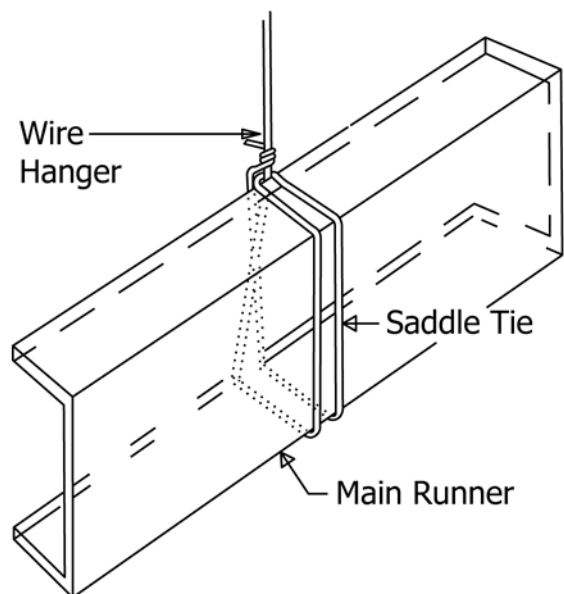
FIG. 3 Saddle-Tie
