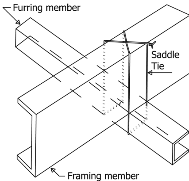
FIG. 2 Saddle-Tie
