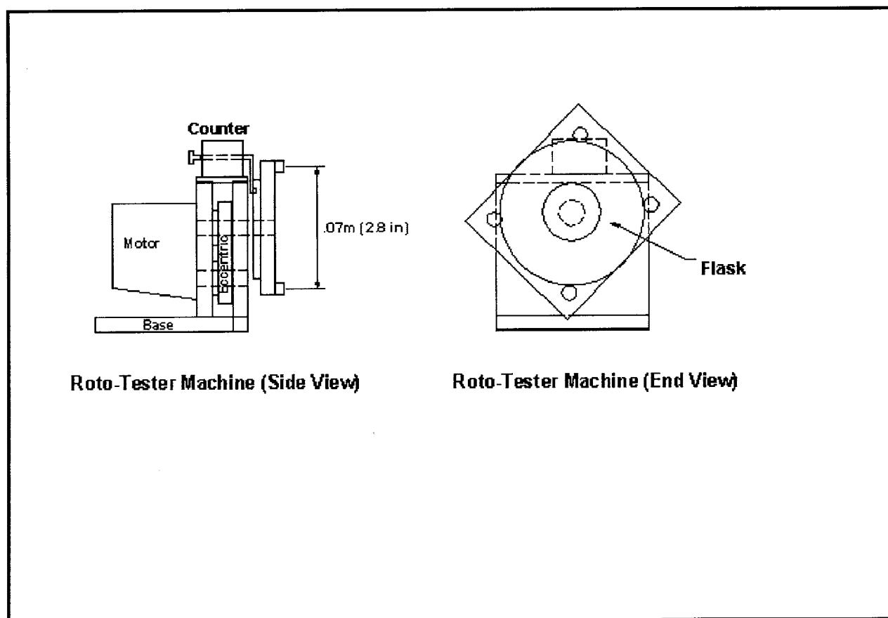
FIG. 2 Roto-Tester
