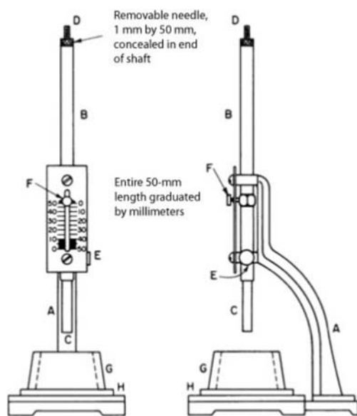
FIG. 1 Vicat Apparatus
