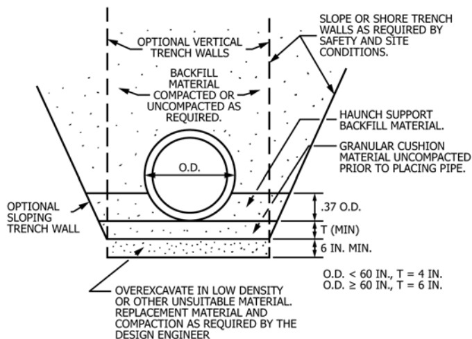
FIG. X1.1 Pipe Bedding
