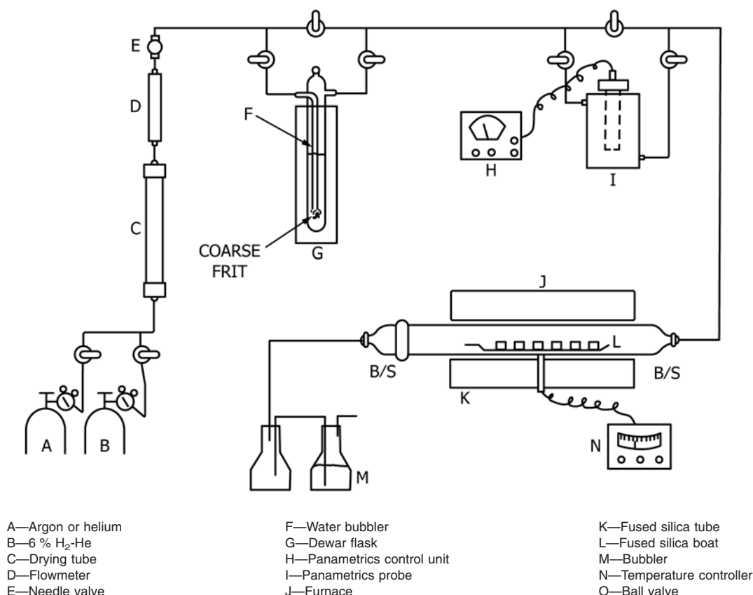
FIG. 10 O/M Apparatus
