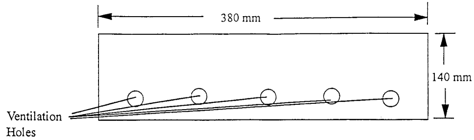
FIG. X1.3 Lid—From Above
