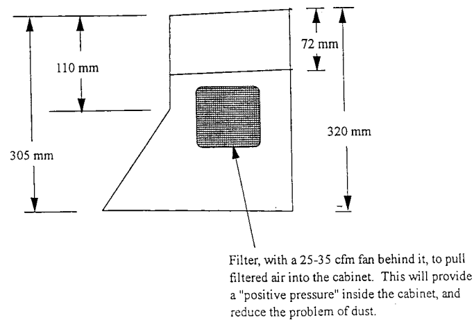
FIG. X1.5 End Elevation
