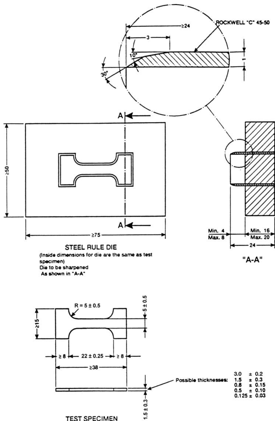
FIG. 1 Microtensile Die and Test Specimen
