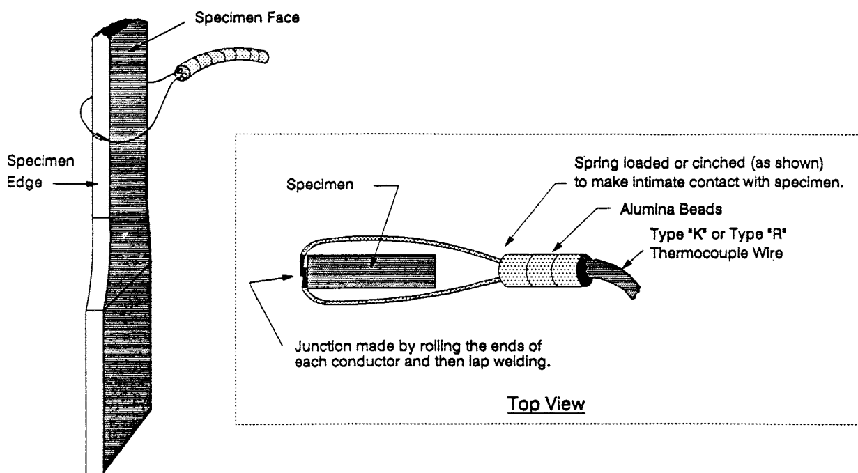
FIG. 6 Wraparound Thermocouple
