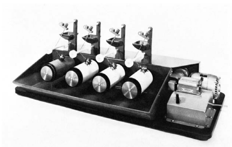
FIG. 1 ICI Mace Tester
