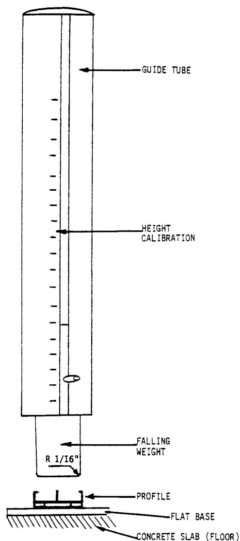
FIG. 2 Testing Apparatus
