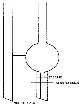
FIG. A3.1 Viscometer Fill Line
