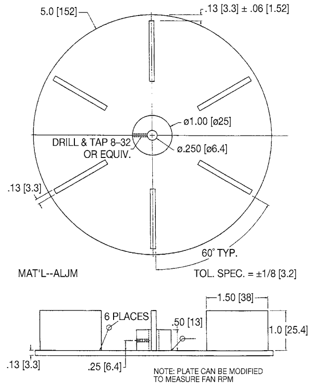
FIG. A1.5 Fan Impeller
