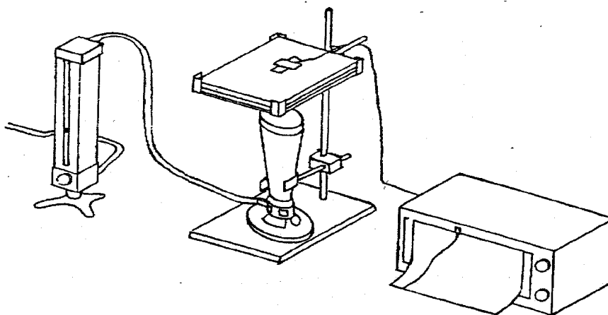
FIG. 1 Test Apparatus
