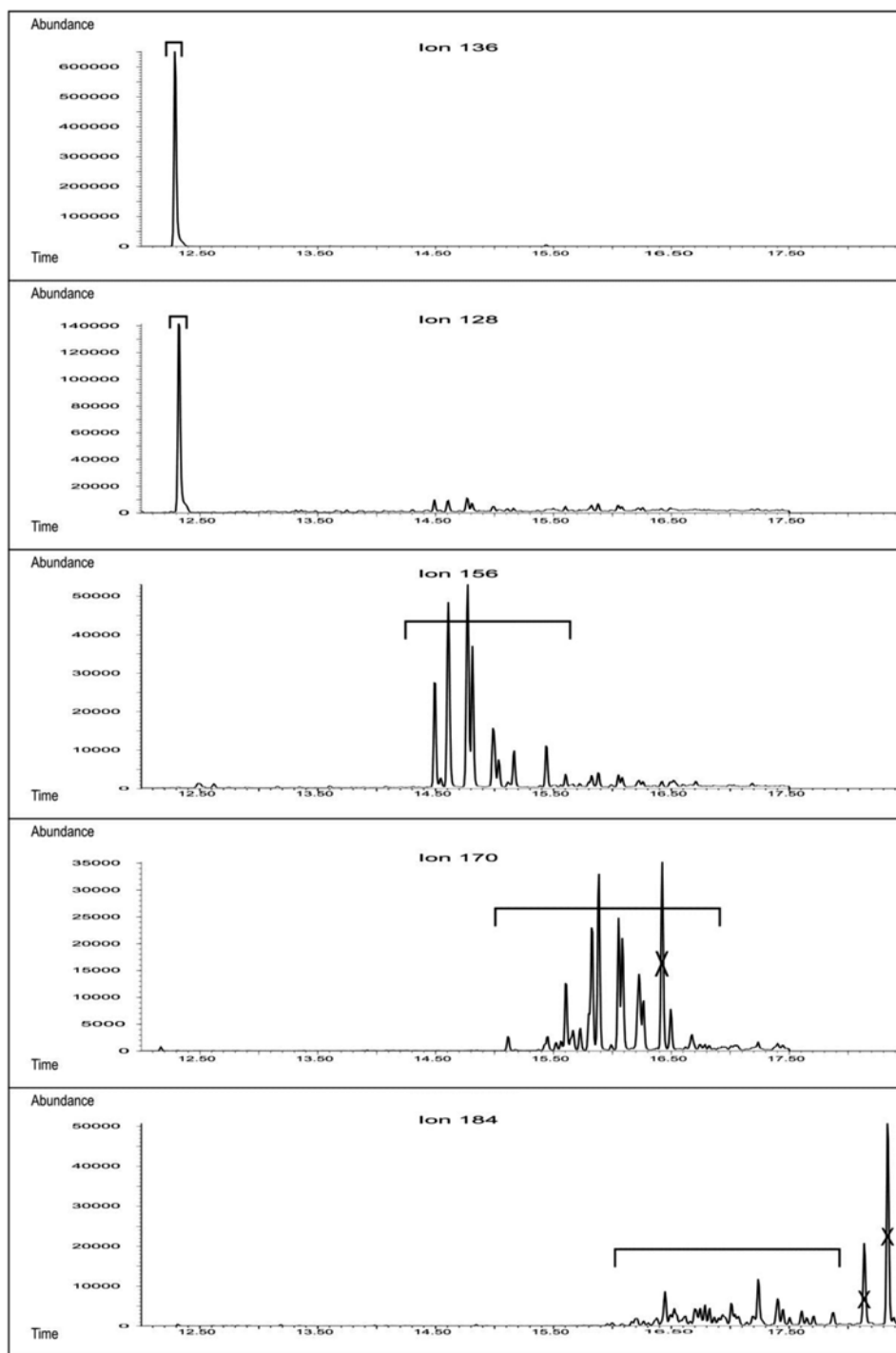
FIG. X1.1 Naphthalenes
