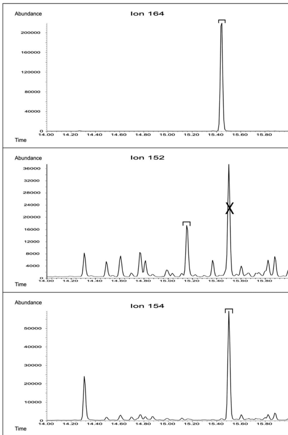
FIG. X1.3 Acenaphthylene/Acenaphthene
