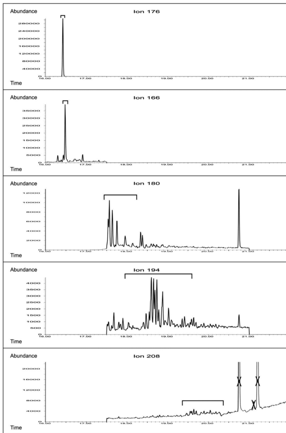
FIG. X1.4 Fluorenes
