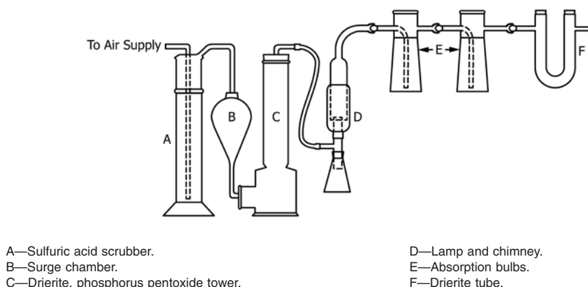
FIG. 2 Apparatus Assembly
