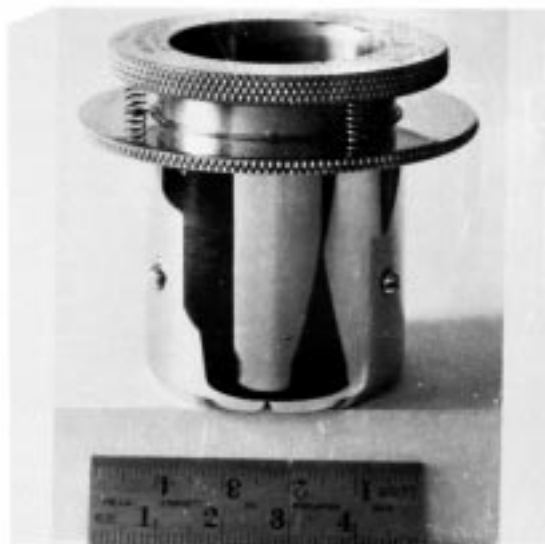
FIG. 3 Pfund Gage
