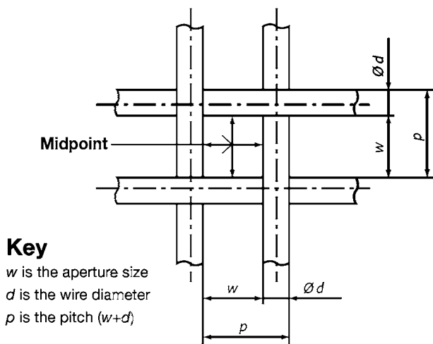
FIG. 1 Aperture Size
