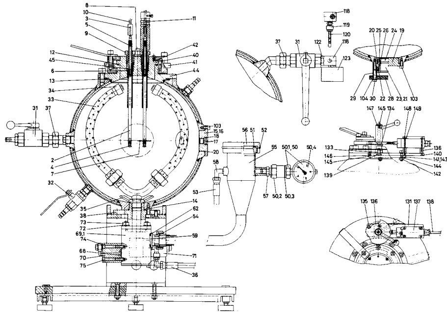
FIG. X1.3 Siwek 20-L Sphere
