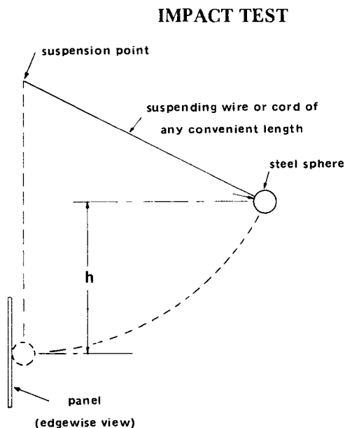
FIG. 7 Impact Test
