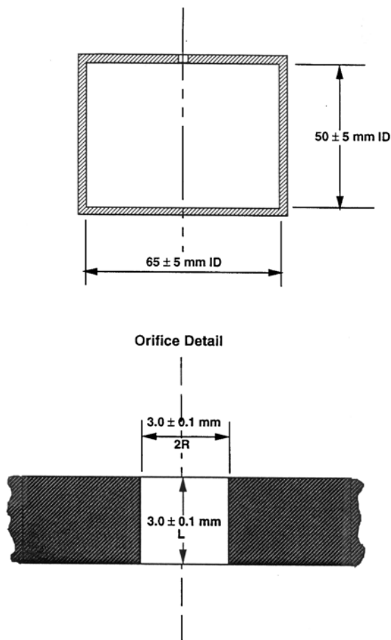
FIG. 4 Effusion Cell
