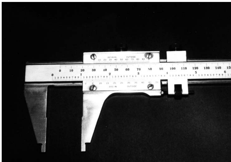
FIG. 13 Vernier Caliper
