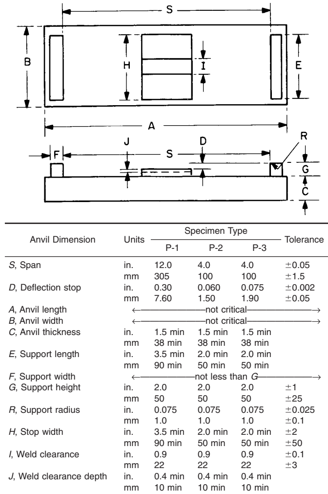
FIG. 4 Anvil Dimensions
