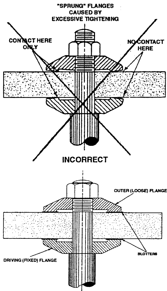
FIG. 4 Spindles
