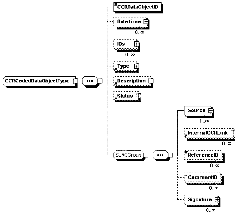
FIG. A2.9 CCRDataObjectID
