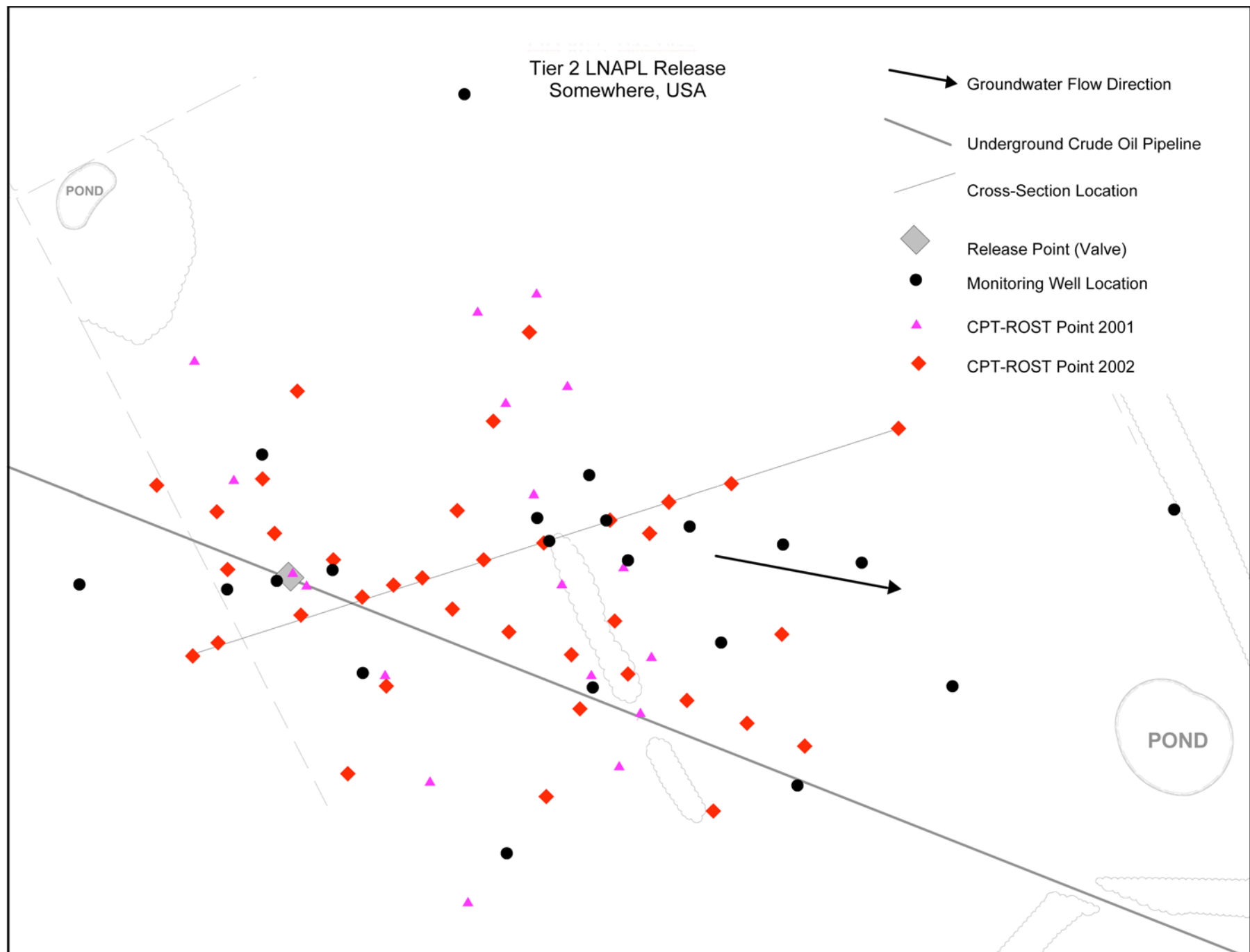
FIG. X6.5 Site Plan
