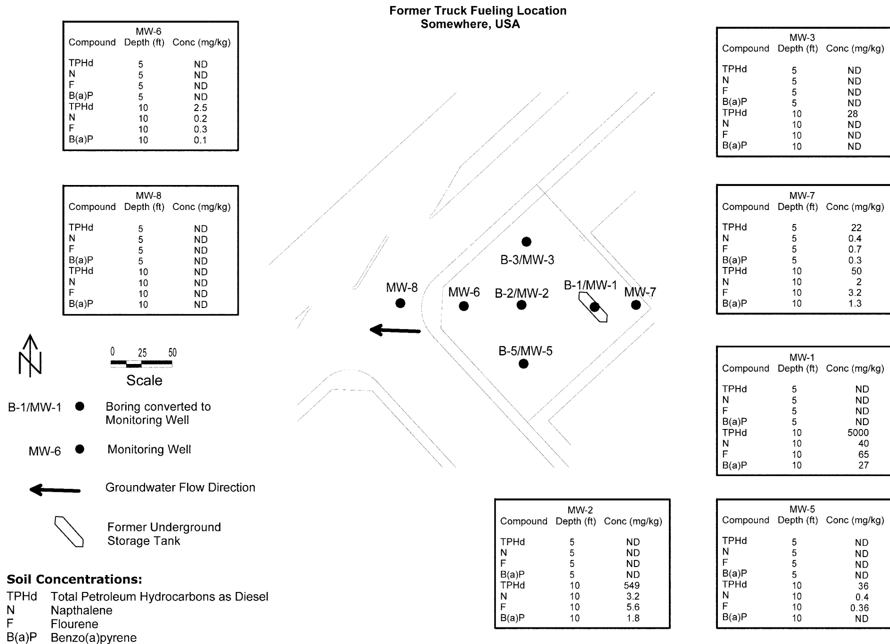
FIG. X6.1 Site Plan
