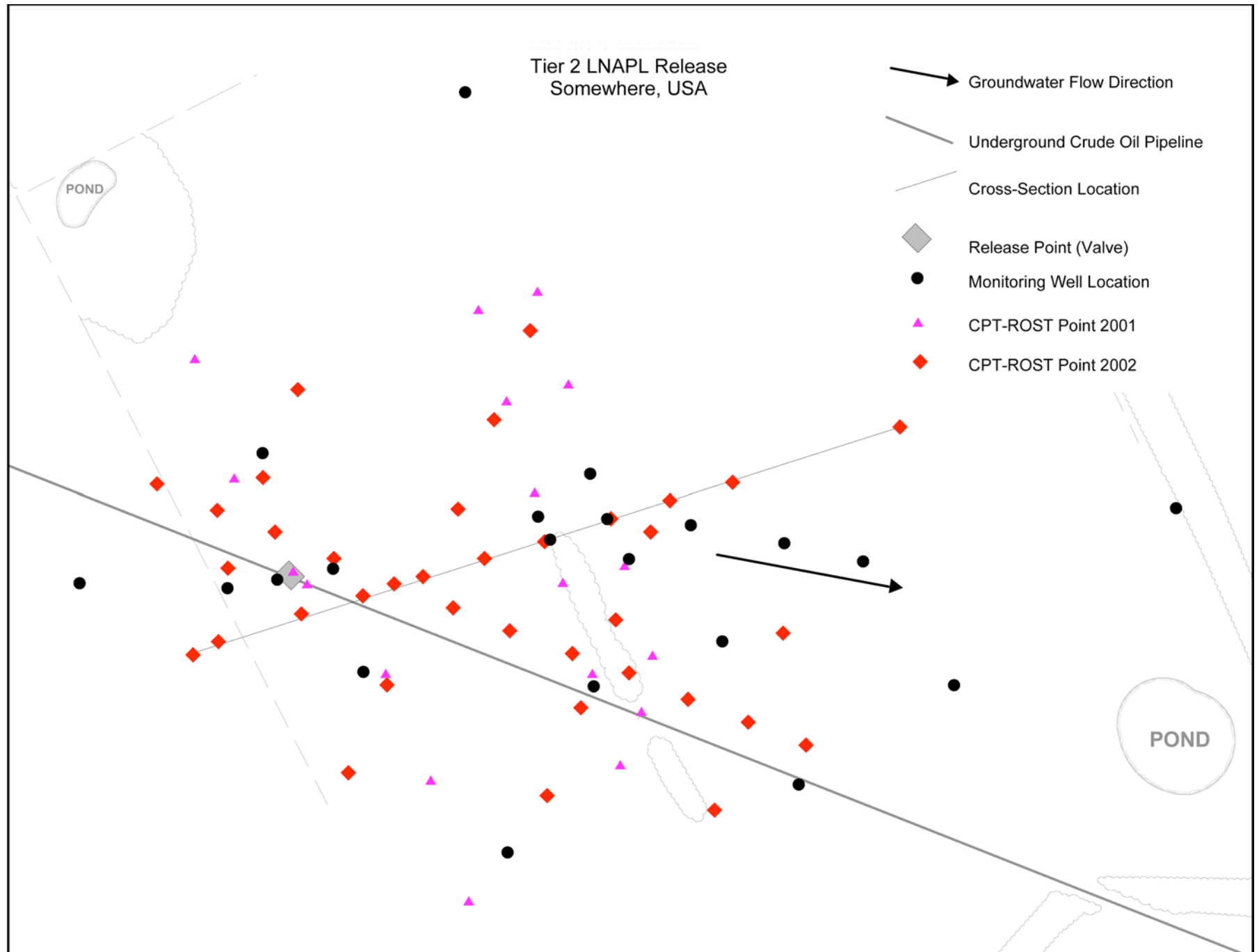
FIG. X6.5 Site Plan
