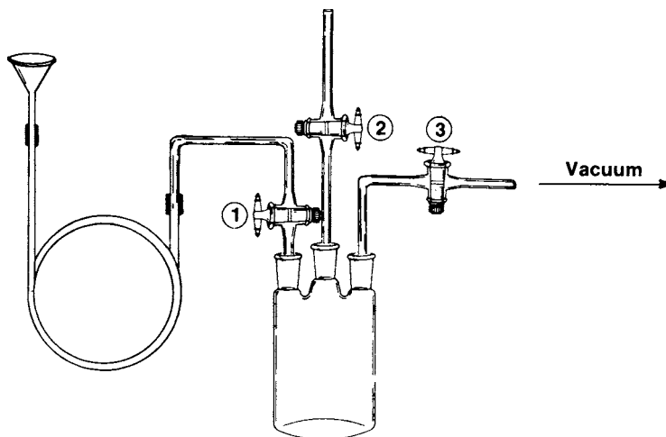
FIG. 2 Vacuum Fill Apparatus
